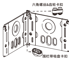
⑥ 将围栏片与围栏片组装
