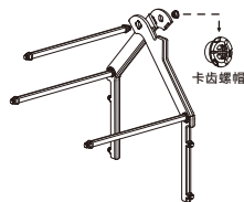
③ 将两边组装好的支架,用支撑杆拼接在一起
