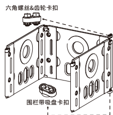
⑦ 将围栏片组装到另一侧
