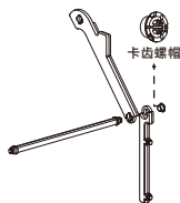
② 拼接另一边A/B型支架,并用支撑杆和卡齿螺帽固定
