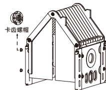
⑨ 用卡齿螺帽将屋顶架与围栏片固定
